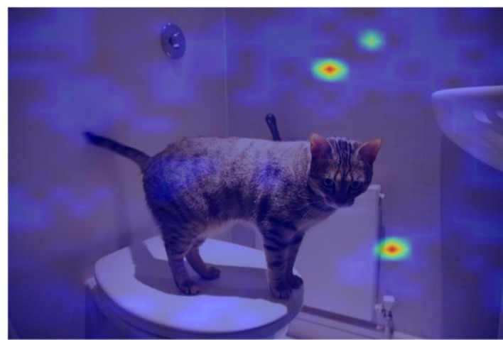
CLIP
