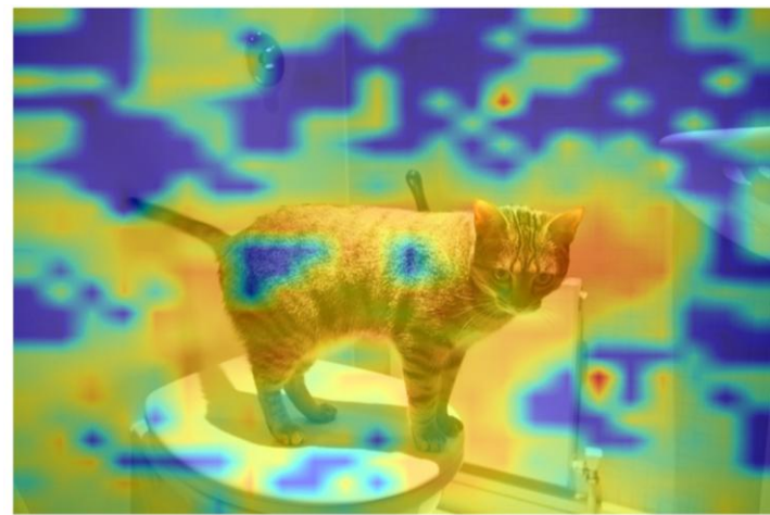
Prompt 2
