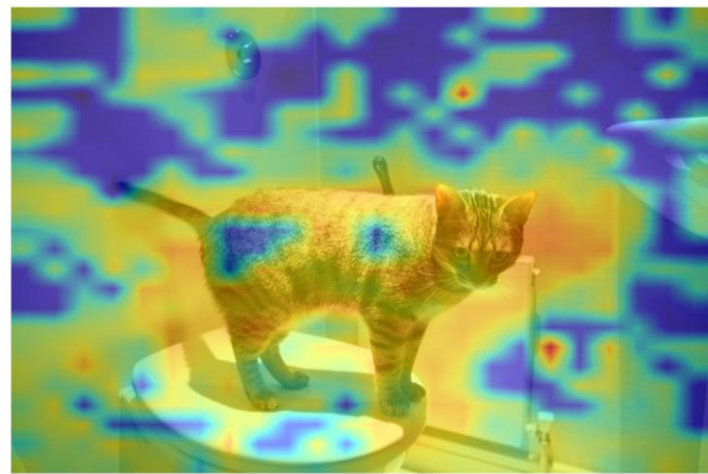
Prompt 1
