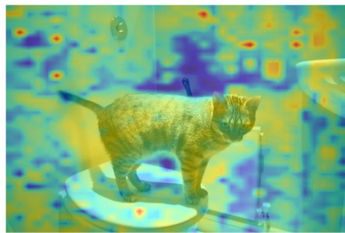
DINOv2
